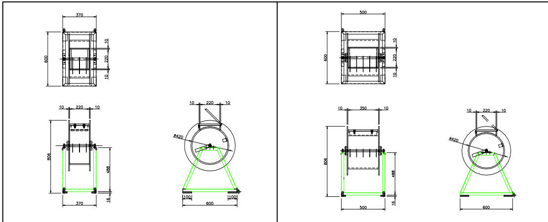
[0.8kg型 形状図]
